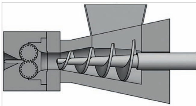
Bild 3: Schematische Darstellung: Konisches Doppelschnecken- Fütteraggregat und Zahnradpumpe
