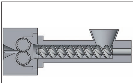
Bild 2: Schematische Darstellung: Einschncken-Fütteraggregat und Zahnradpumpe
